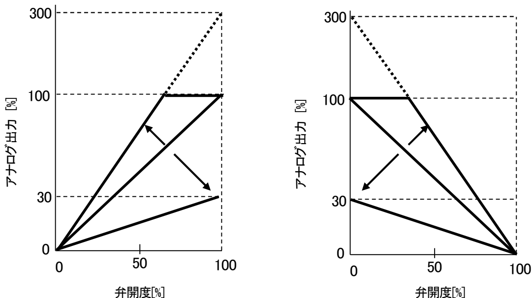
(a) 弁開度増加でアナログ出力増加
