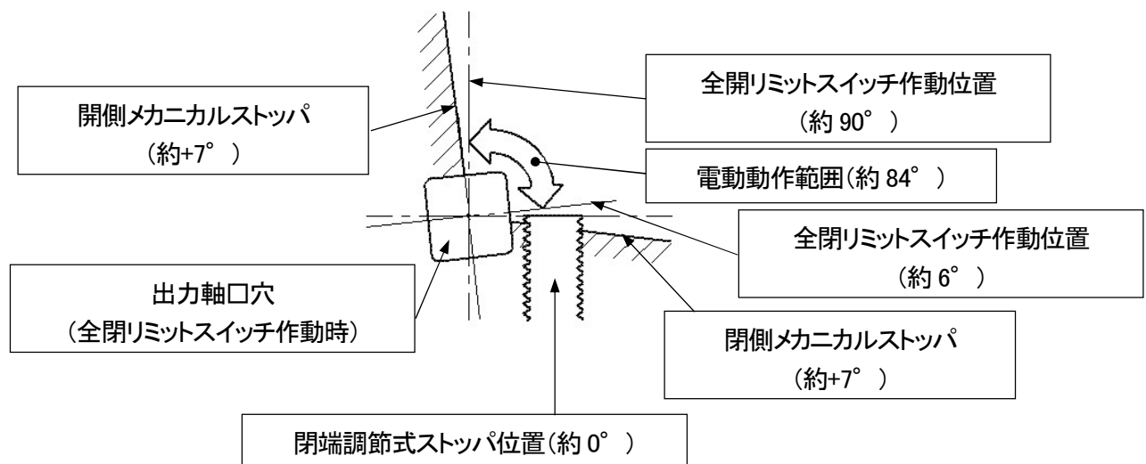
図 付 1-1 リミットスイッチ動作位置
