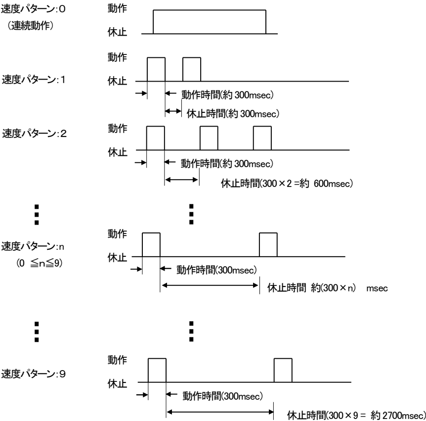
図 9-13(a) 速度パターン
