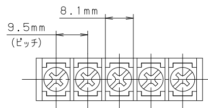
図 1-11(b) 端子寸法
