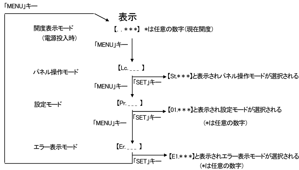
図 9-2 各モードの切替え
