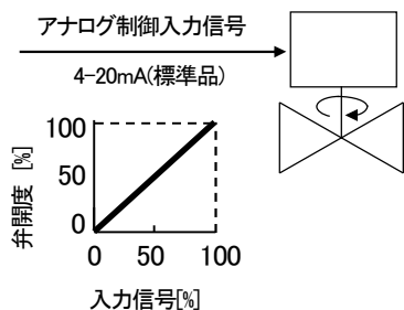
図 8-1 比例制御(逆作動)
