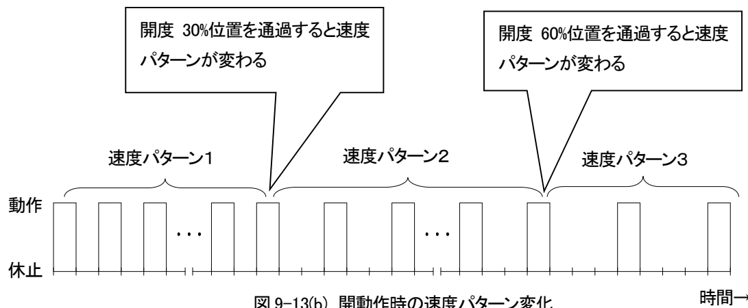
図 9-13(b) 開動作時の速度パターン変化
