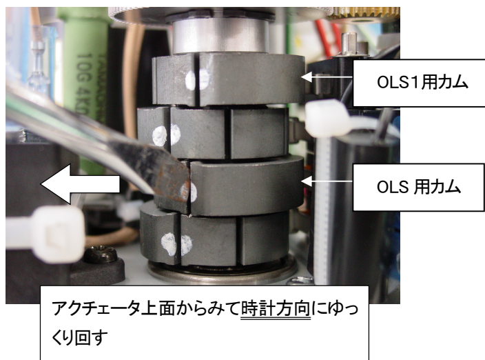
図 12-12 OLS、OLS1 調整
