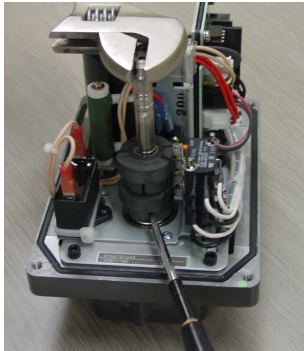
図 12-13(b) 閉側カム調整
