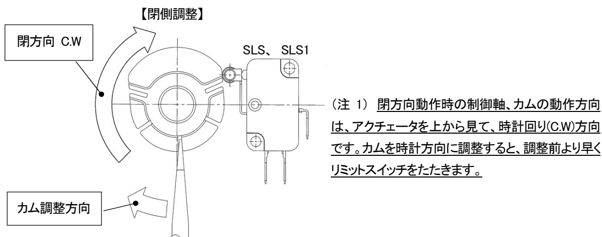
図 12-8(a) 閉側カム調整
