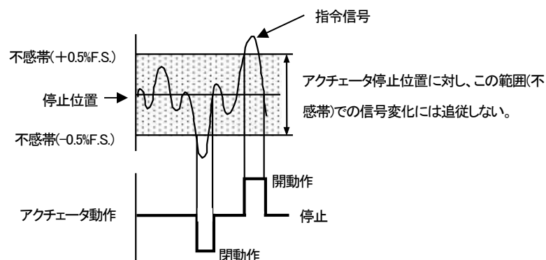
図 9-4 不感帯
