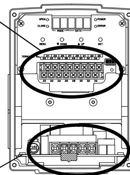
図 1-9 基板各部配置図
