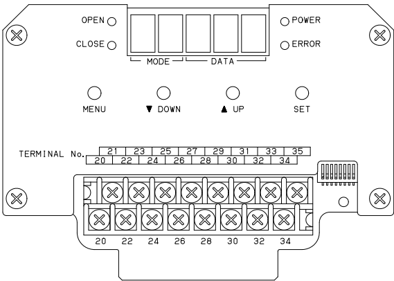
図 9-1 操作パネル
