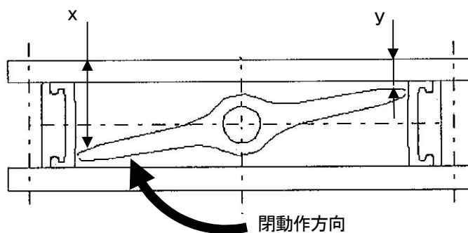
図 12-5 DJ 型バタフライ弁全閉位置
