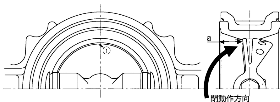
図 12-4 HRDJ 型バタフライ弁全閉位置
