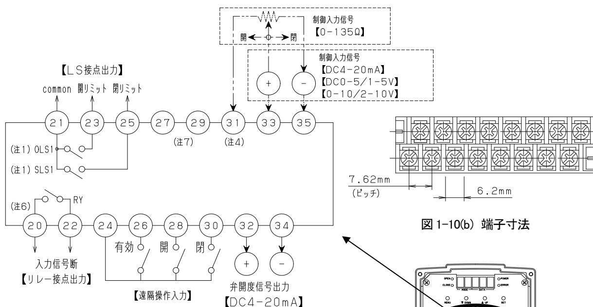
図 1-10(a) 制御用端子配線図
