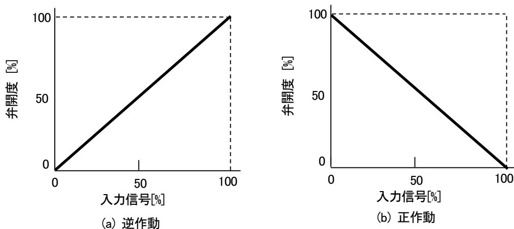
図 9-6 バルブ動作
