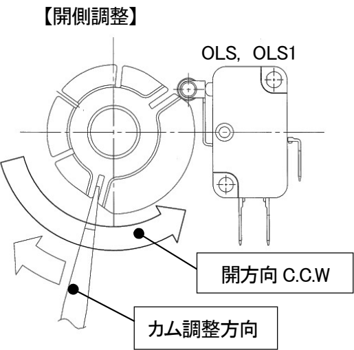
図 12-13(a) 開側カム調整
