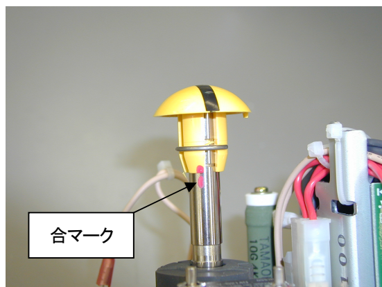
図 12-16 合マーク
