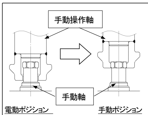
図 12-2 手動操作機構詳細図
