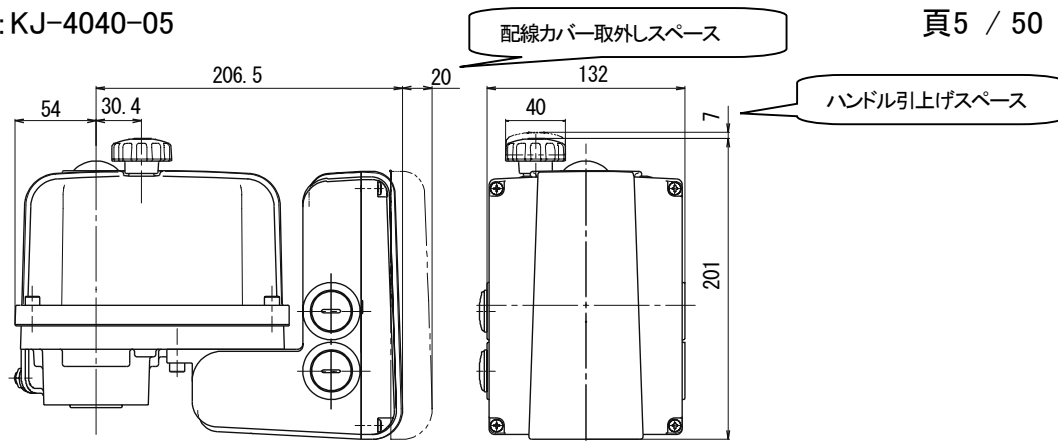
図 1-4 EXCN100/200-2 外観図
