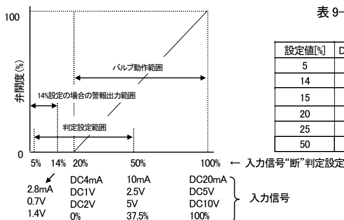
図 9-5 入力信号“断”判定動作
