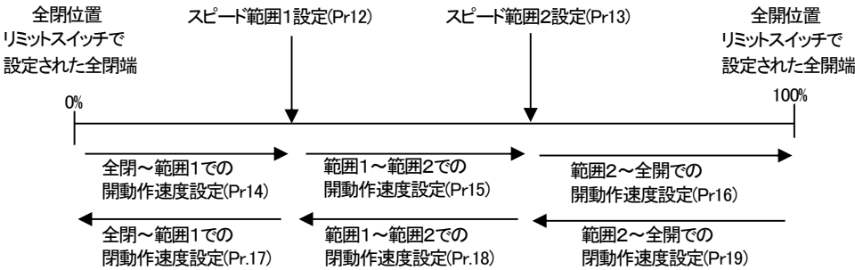
図 9-12 スピード設定
