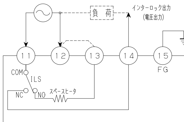
図 1-11(a) 電源用端子配線図
