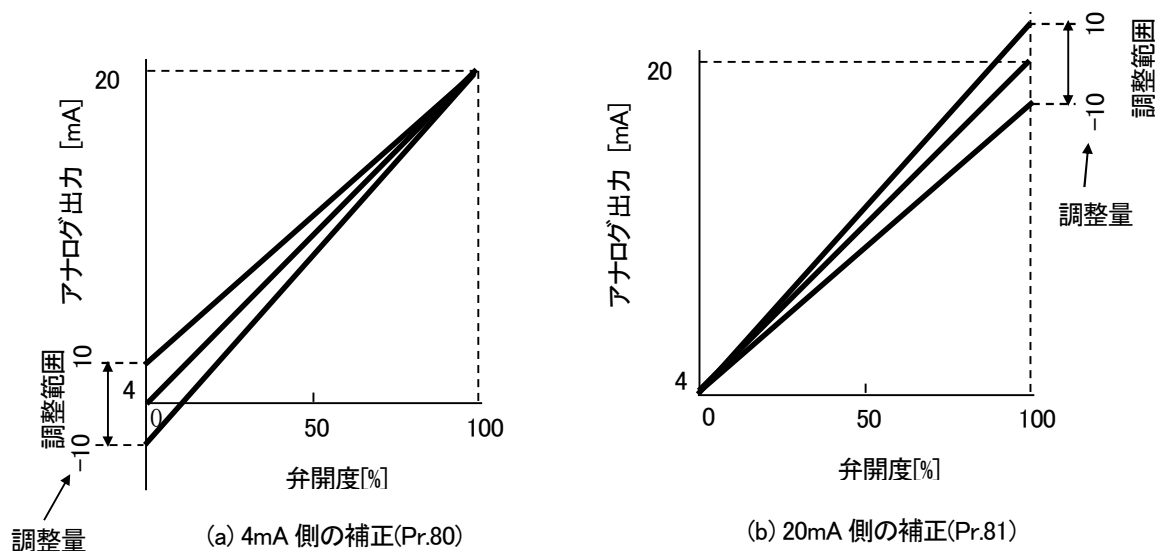
図 9-14 アナログ出力補正
