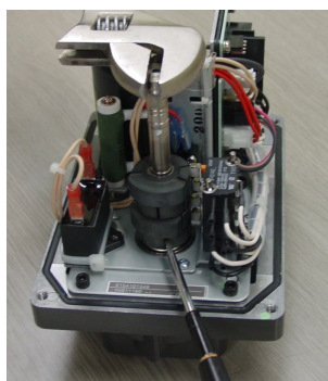
図 12-8(b) 閉側カム調整
