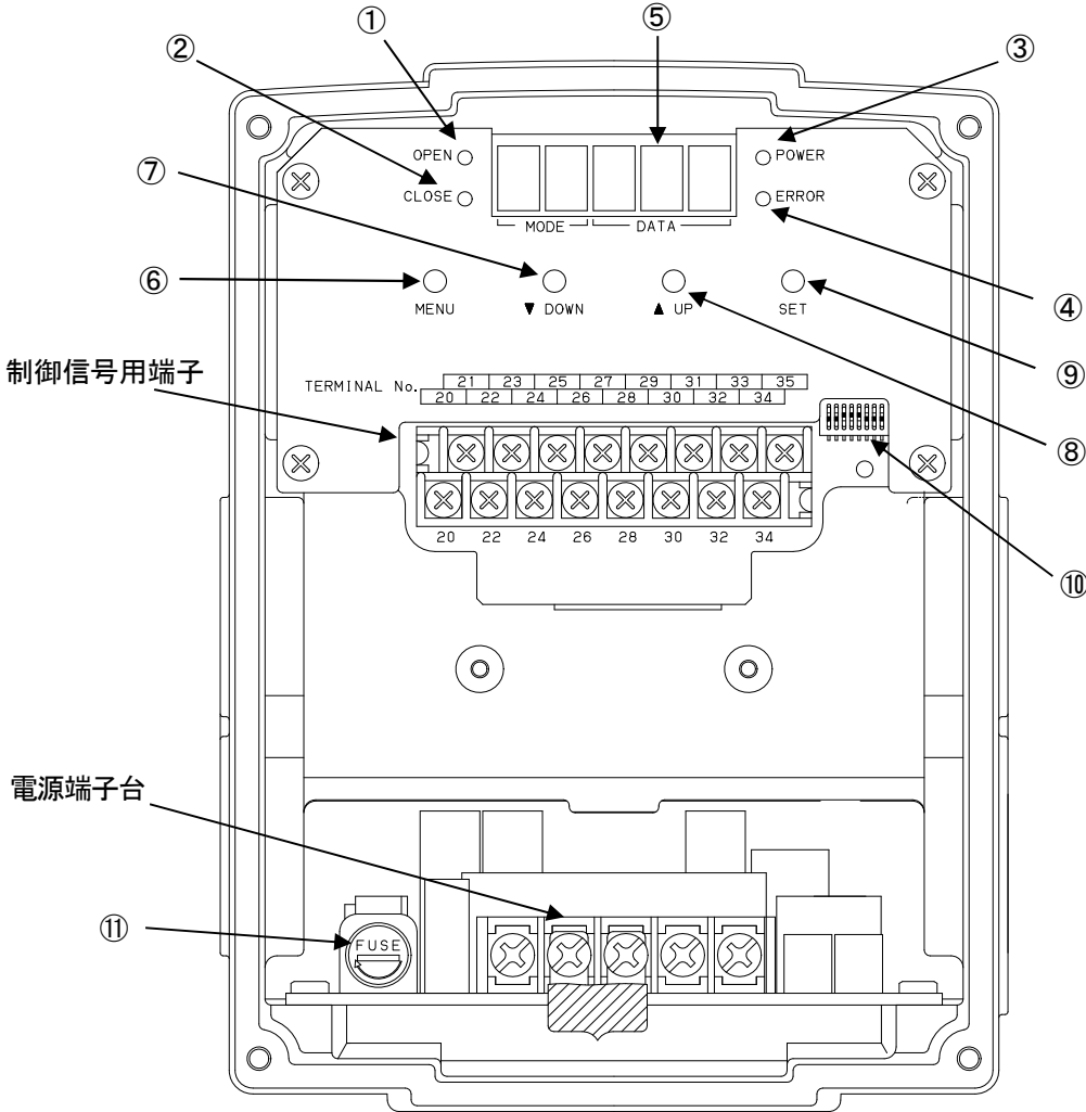
図 1-8 基板各部配置図
