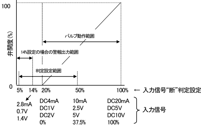
図 1-2 制御動作図
