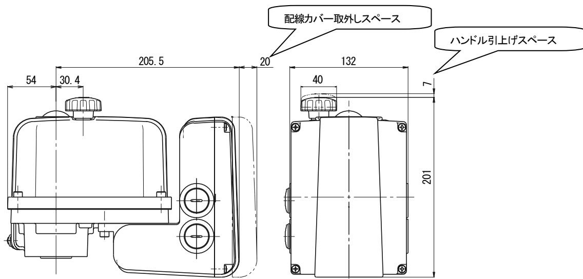
図 1-4 EXCN100/200-2 外観図
