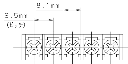
図 1-10(b) 端子寸法
