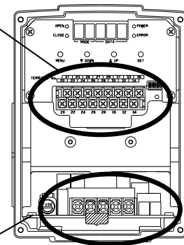
図 1-8 基板各部配置図
