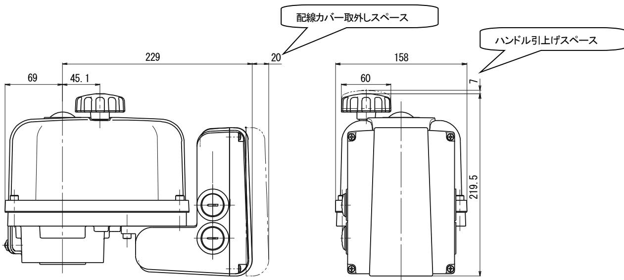
図 1-5 EXCN100/200-3 外観図
