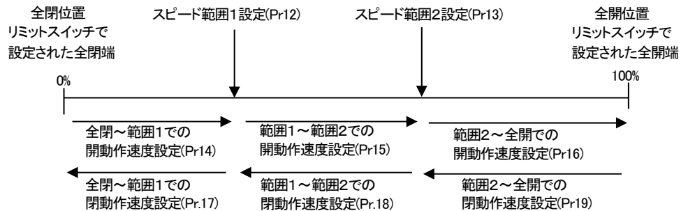
図 9-12 スピード設
