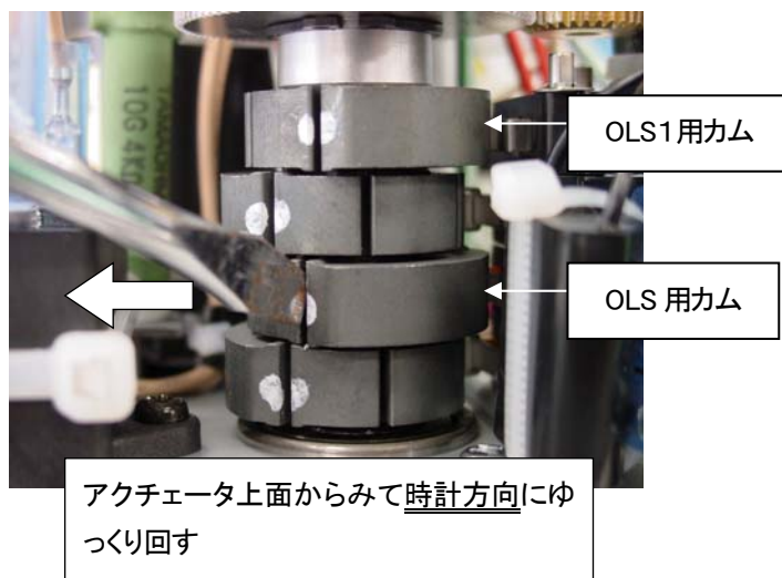
図 12-12 OLS、OLS1 調整
