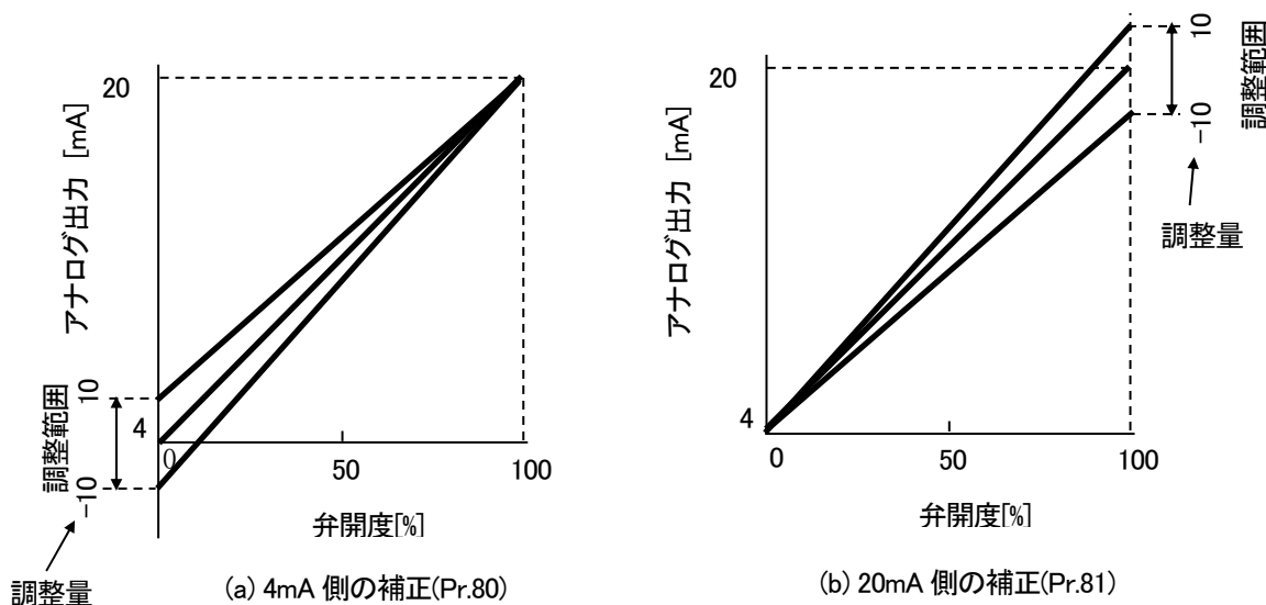
図 9-14 アナログ出力補正
