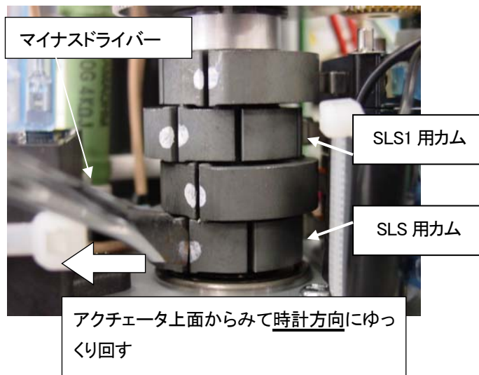
図 12-7 SLS、SLS1 調整
