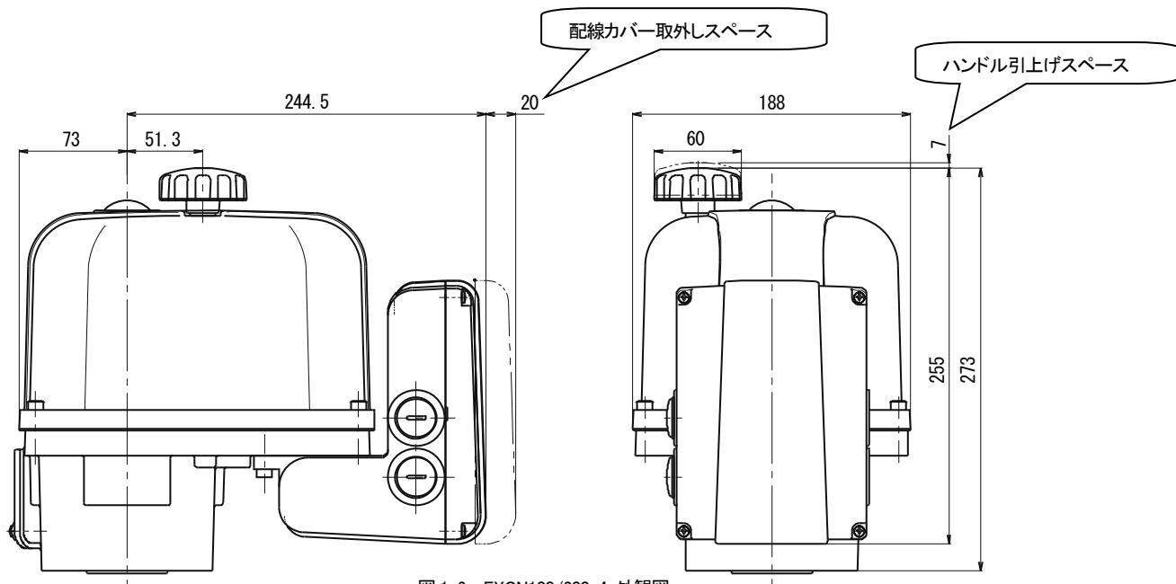
図 1-6 EXCN100/200-4 外観図
