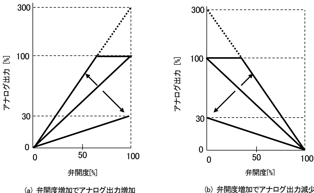
図 9-11 アナログ出力傾き調整
