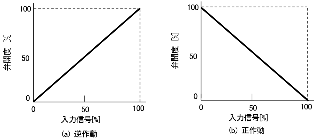
図 9-6 バルブ動作
