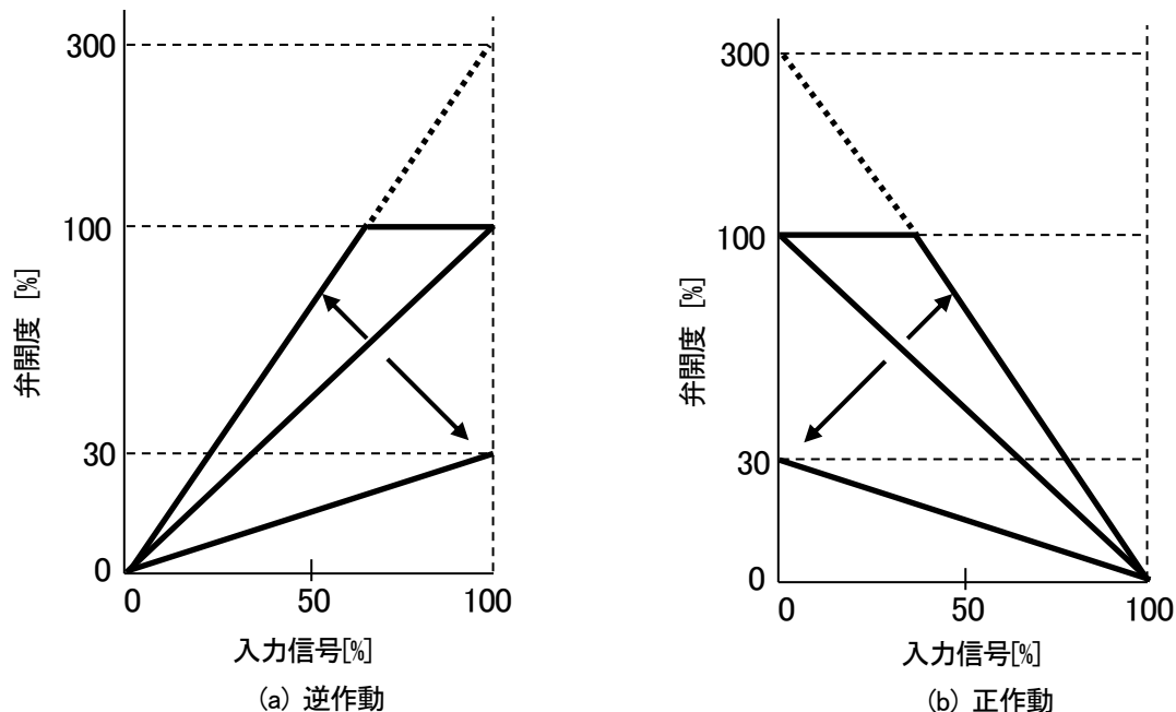
図 9-8 アナログ入力傾き調節
