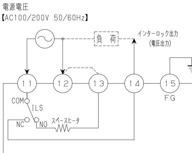
図 1-10(a) 電源用端子配線図
