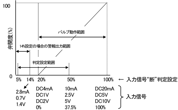
図 1-2 制御動作図
