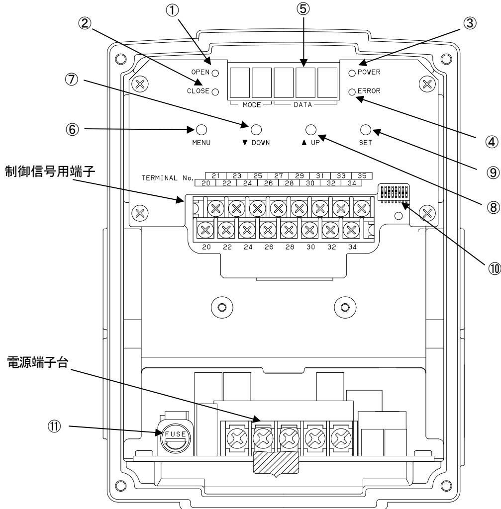
図 1-7 基板各部配置図
