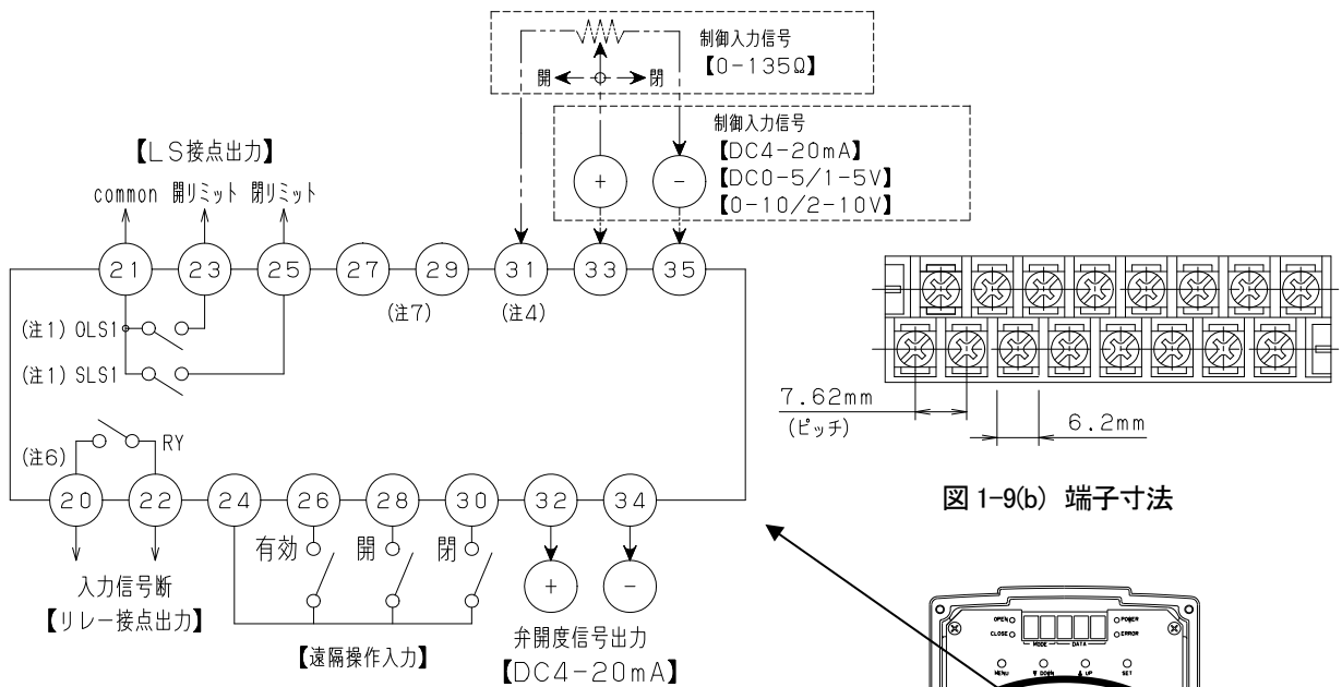
図 1-9(a) 制御用端子配線図
