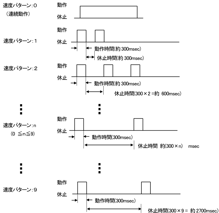
図 9-13(a) 速度パターン
