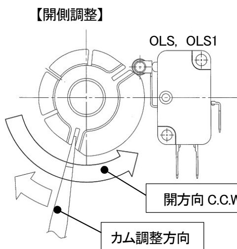
図 12-13(a) 開側カム調整
