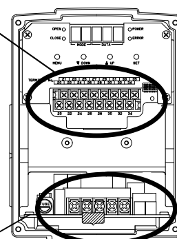
図 1-10 基板各部配置図
