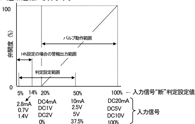
図 1-2 制御動作図
