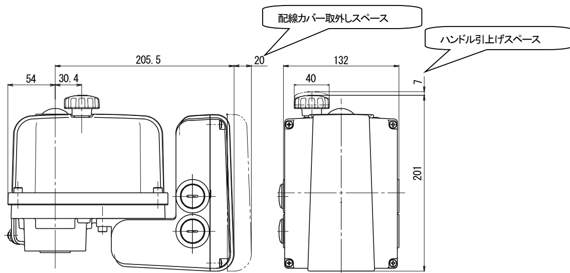
図 1-5 EXD100/200-2 外観図
