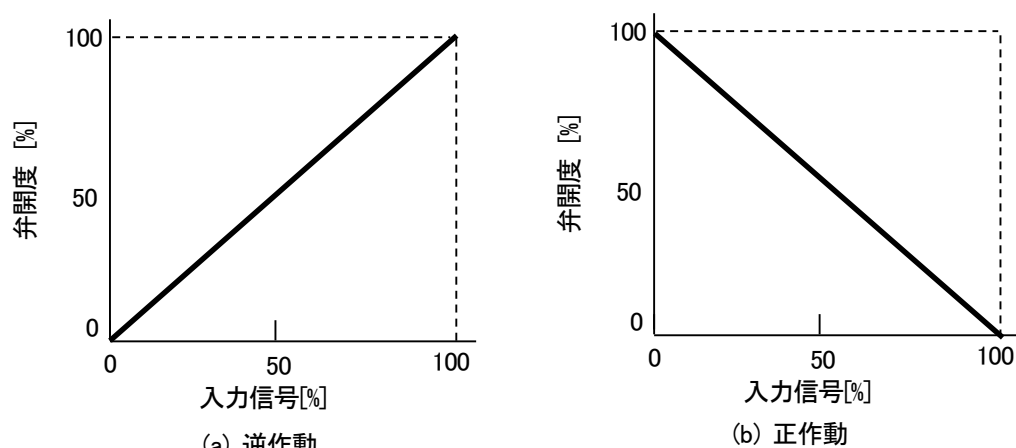
図 9-6 バルブ動作
