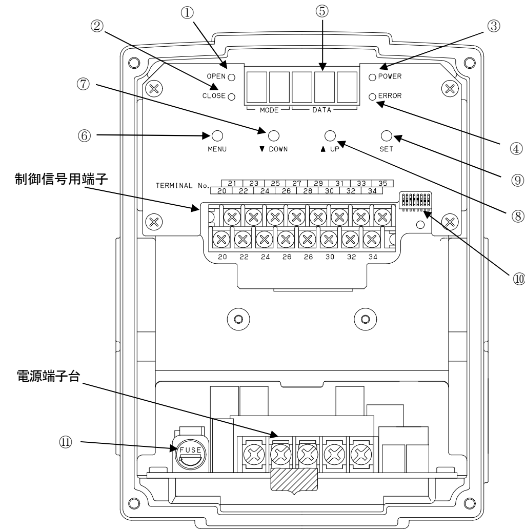
図 1-8 基板各部配置図
