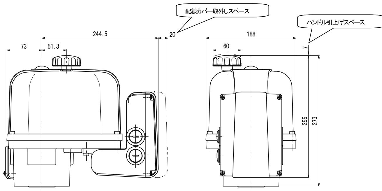
図 1-7 EXD100/200-4 外観図
