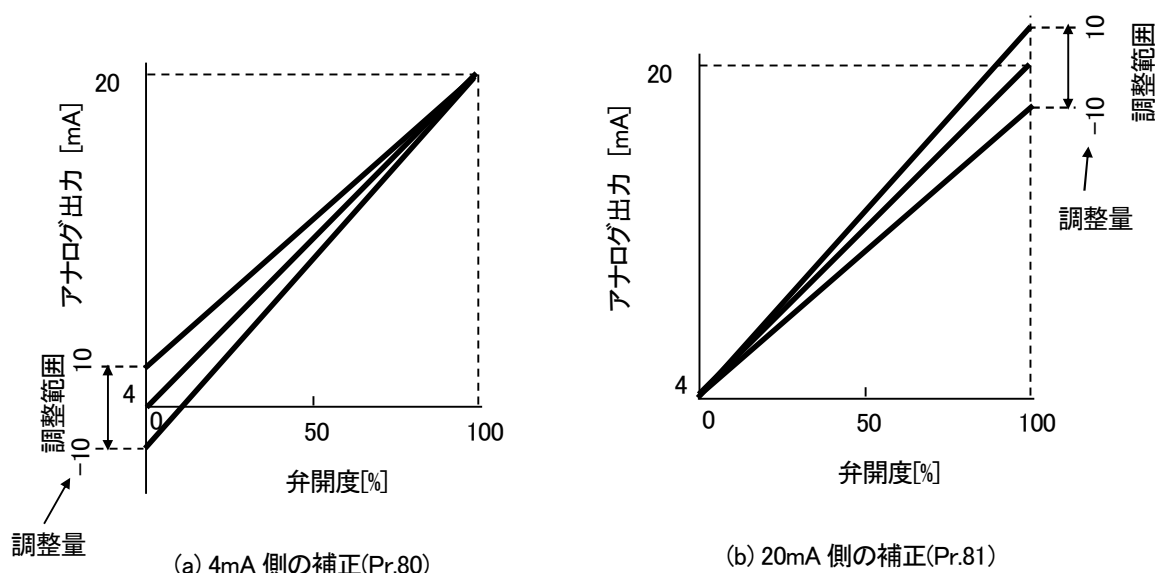
図 9-15 アナログ出力補正
