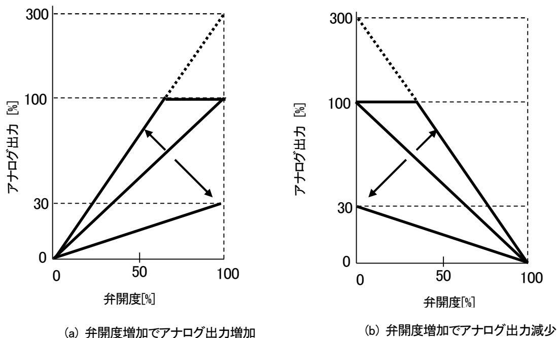
図 9-11 アナログ出力傾き調整
