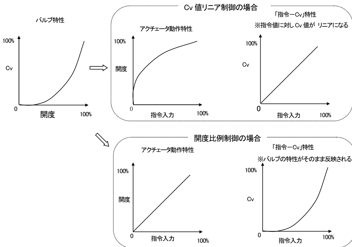
図 8-4 Cv リニア制御と開度比例制御
