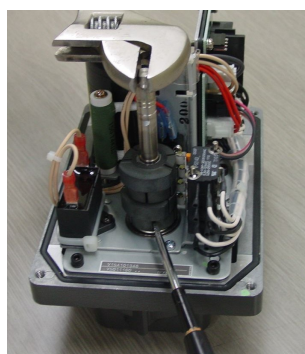
図 12-13(b) 閉側カム調整
