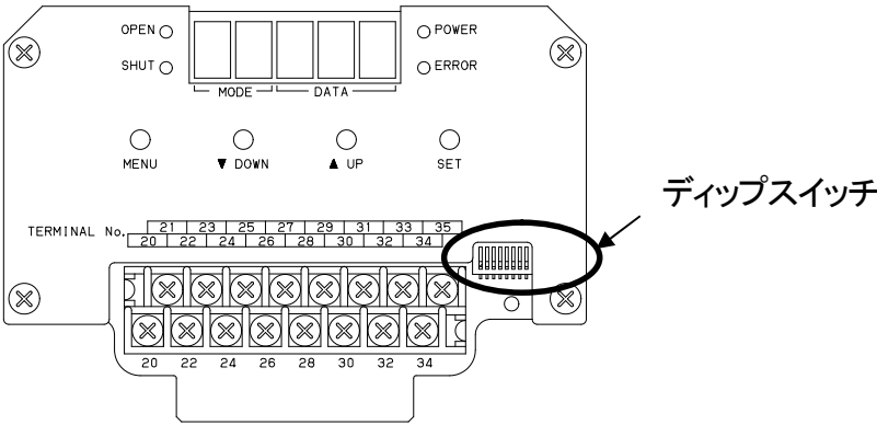
図 13-1 ディップスイッチの位置
