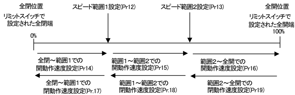
図 9-13 スピード設定
