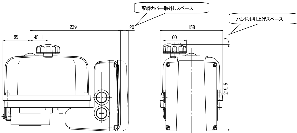
図 1-6 EXD100/200-3 外観図
