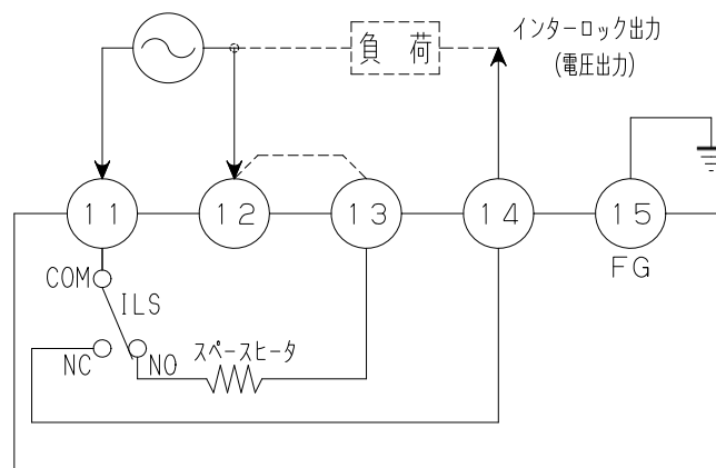
図 1-11(a) 電源用端子
