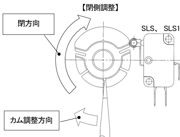
図 12-8(a) 閉側カム調整
