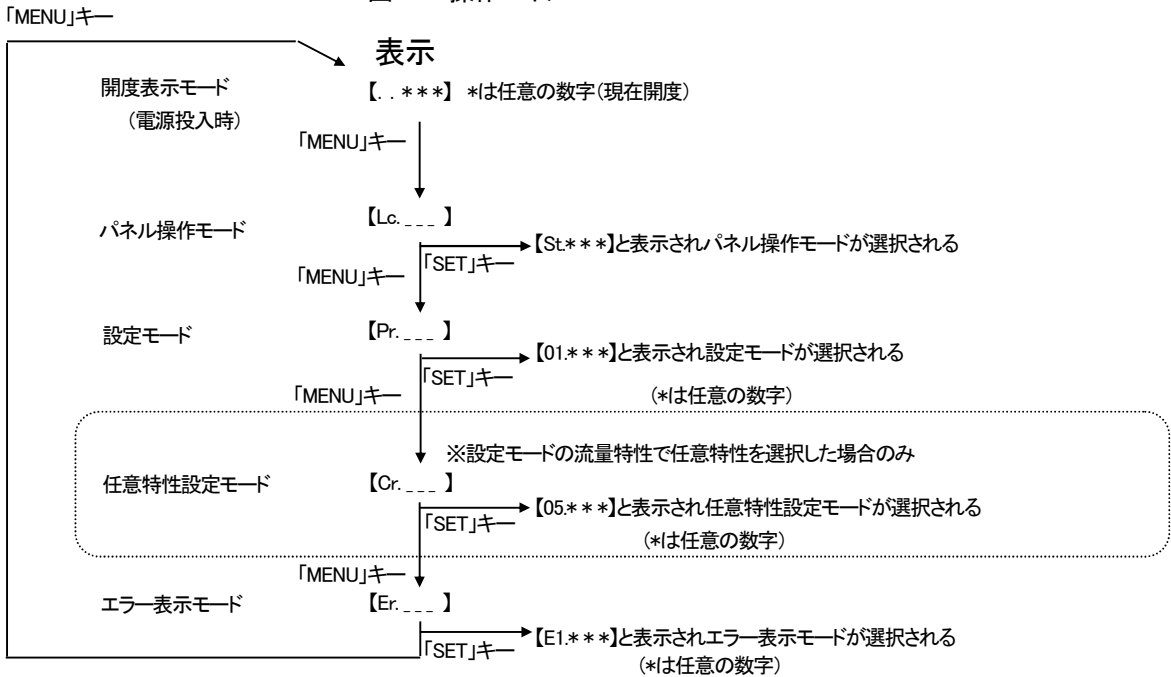
図 9-2 各モードの切替え
