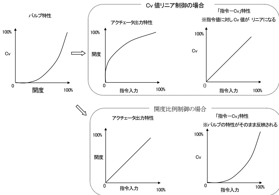
図 1-3 Cv リニア制御と開度比例制御
