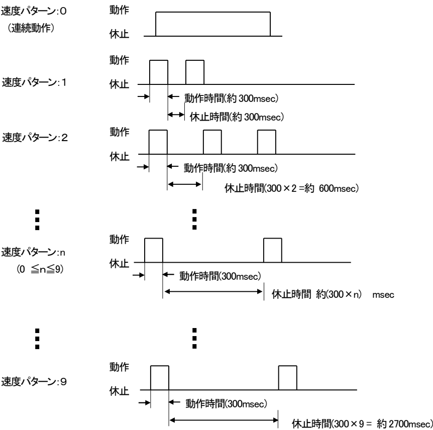
図 9-14(a) 速度パターン
