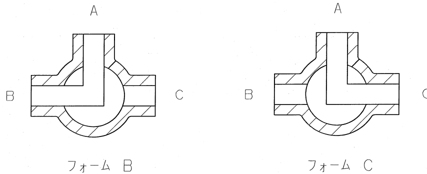
図 15 横三方ボールバルブ 流路図 (アクチュエータ上部から見て)
