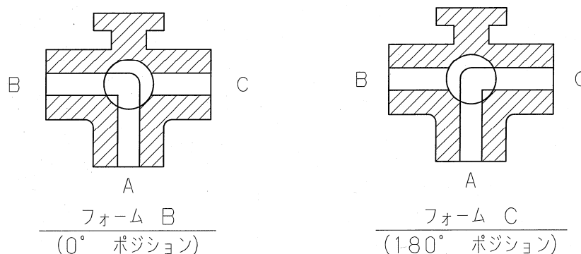
図 16 縦三方ボールバルブ 流路図 (バルブ本体”KITZ“鑄出し文字を表に見て)
