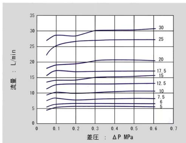
流量特性
