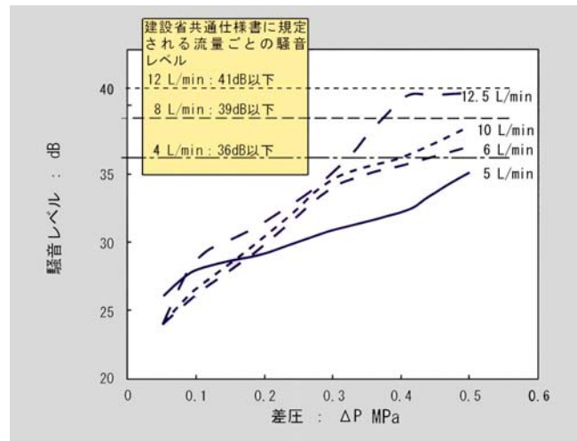
騒音特性
