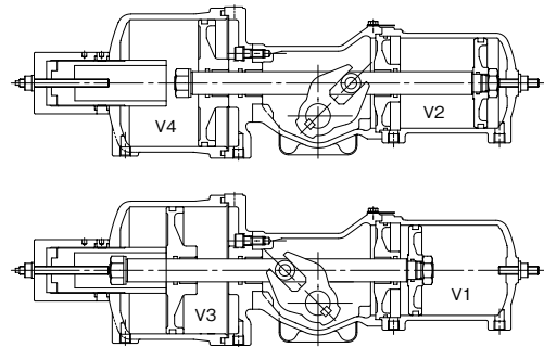
複作動型
