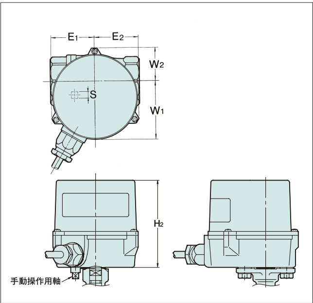
2型寸法表
