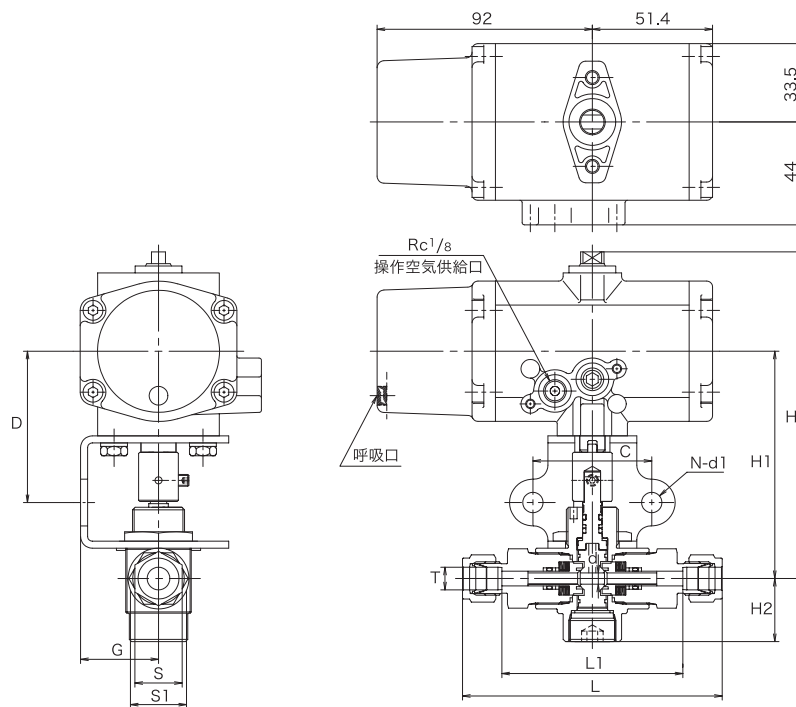
■寸法表
