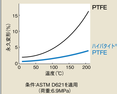
図2 永久変形の温度による変化
