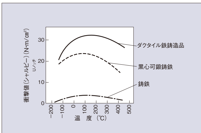
■衝撃値温度特性曲線
