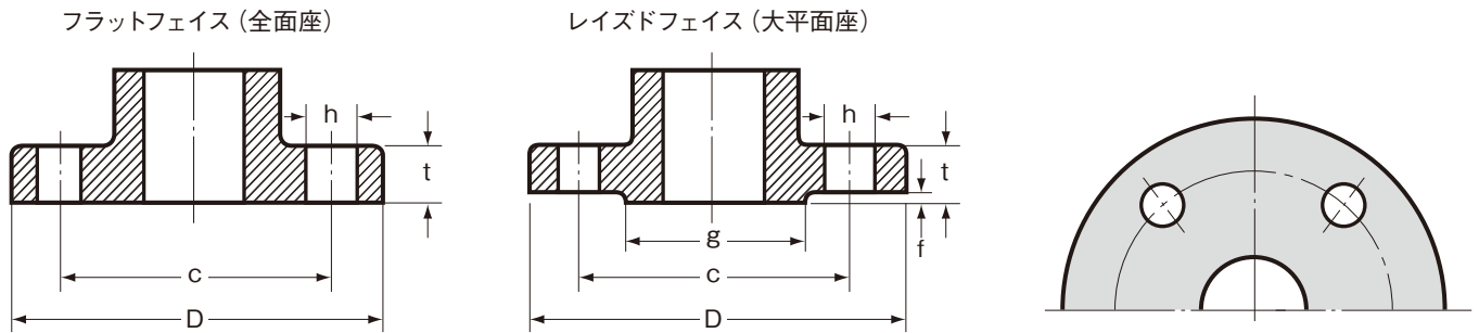
呼び圧力10Kフランジの基準寸法
