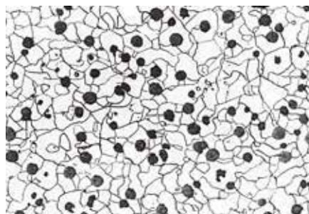
ダクティル鋳鉄
