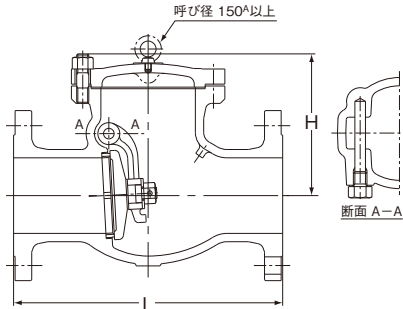
面間寸法：JIS B 2002 フランジ規格：JIS B 2239
