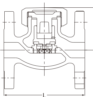
面間寸法：JIS B 2002・JIS B 2051 フランジ規格：JIS B 2239
