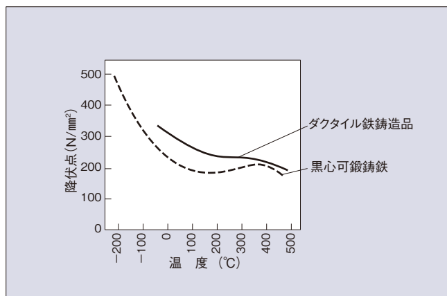
■降伏点温度特性曲線
