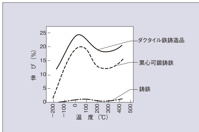
■伸び-温度特性曲線
