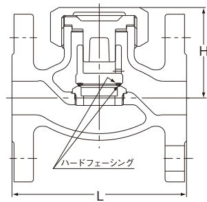
面間寸法：JIS B 2002・JIS B 2051 フランジ規格：JIS B 2239
