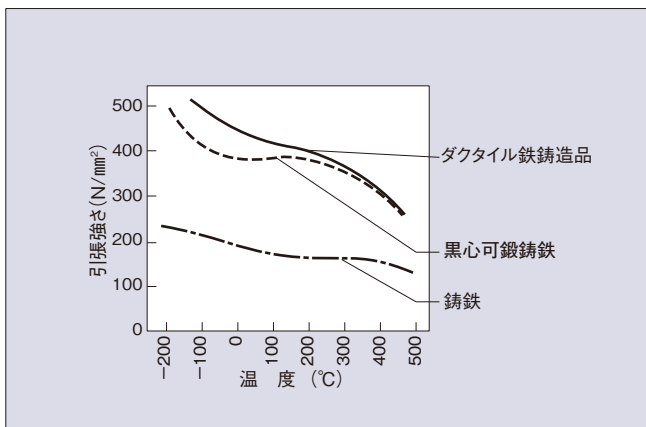
■引張強さ温度特性曲線
