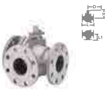
横形三方ボール(SCS13A)
