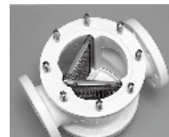
内部構造
