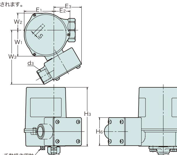
2型寸法表
