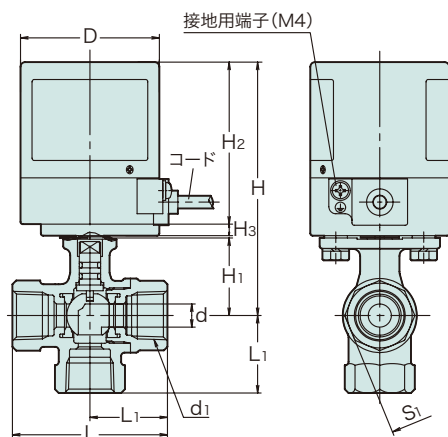
1型・1.5型
