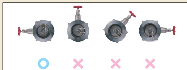
図③水平配管でのバルブ取付姿勢(シングルプレート形)
