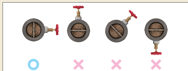
図③水平配管でのバルブ取付姿勢(シングルプレート形)
