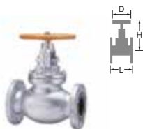
LPガス用グローブ
