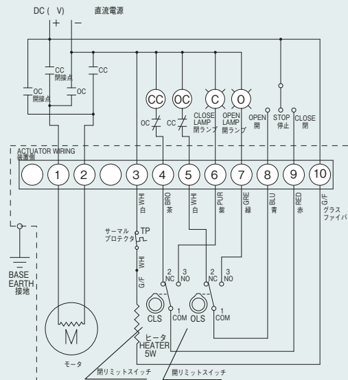
ESHEP*-1 標準 DC電源
