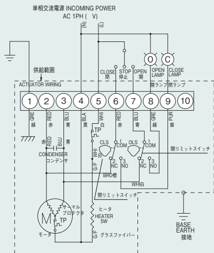
ESHEP*-1 標準 AC電源
