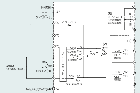
ポテンショメータおよびリレー付の場合
