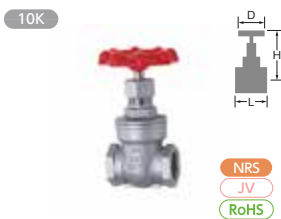
ゲート (SCS13A)
